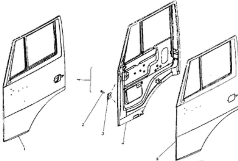
Рис. 238. Дверь левая (сварка) 5320-6100015
