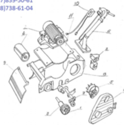
Рис.1. Устройство машины СО-206
